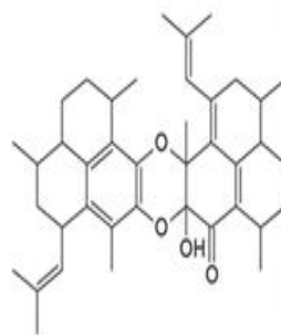
Biselisabethoxane B
